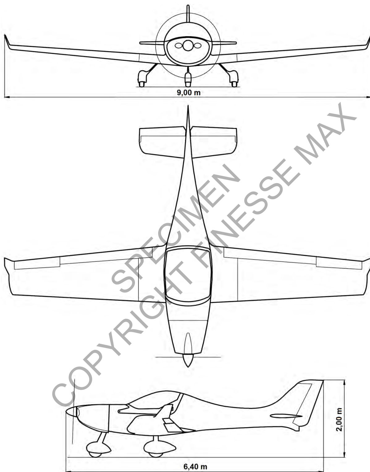
Fig. 1.5-1 Plan 3 vues
