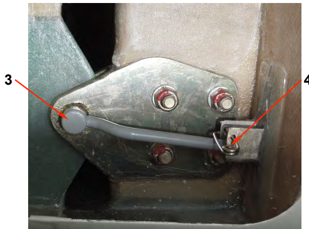
Fig. 4.2-4 Axe auxiliaire (3)
