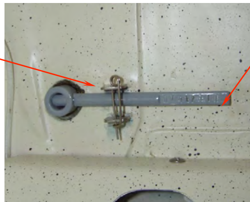
Fig. 4.2-3 Axe intérieur (2)
