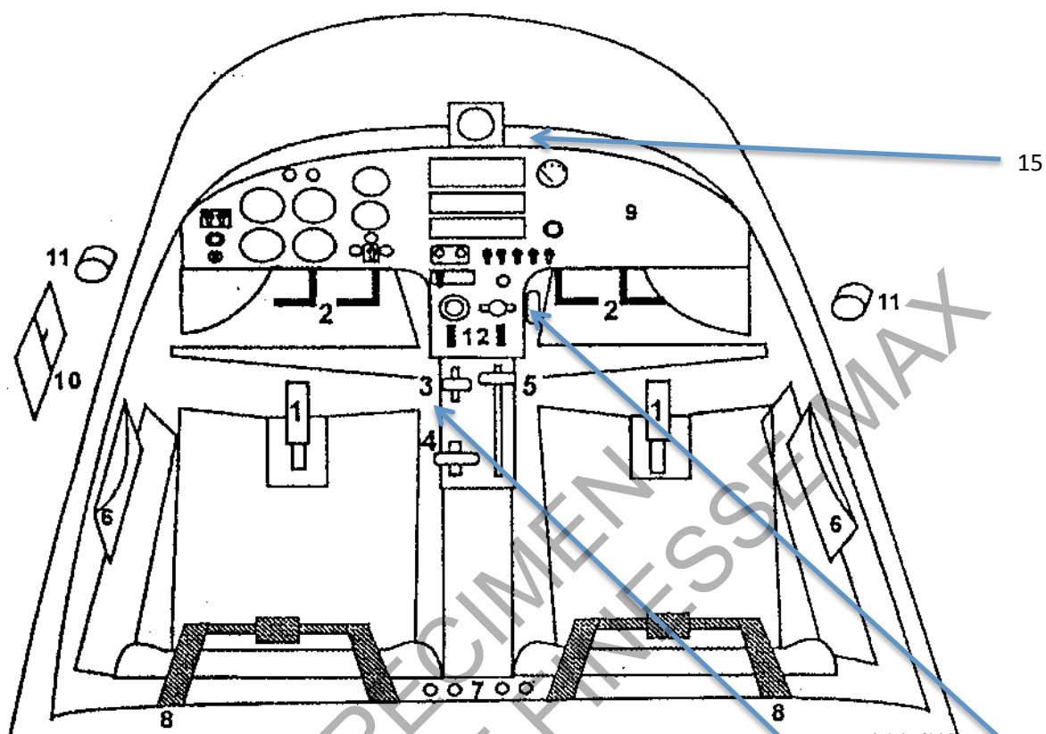
Fig. 4.5-1 Disposition des commandes
