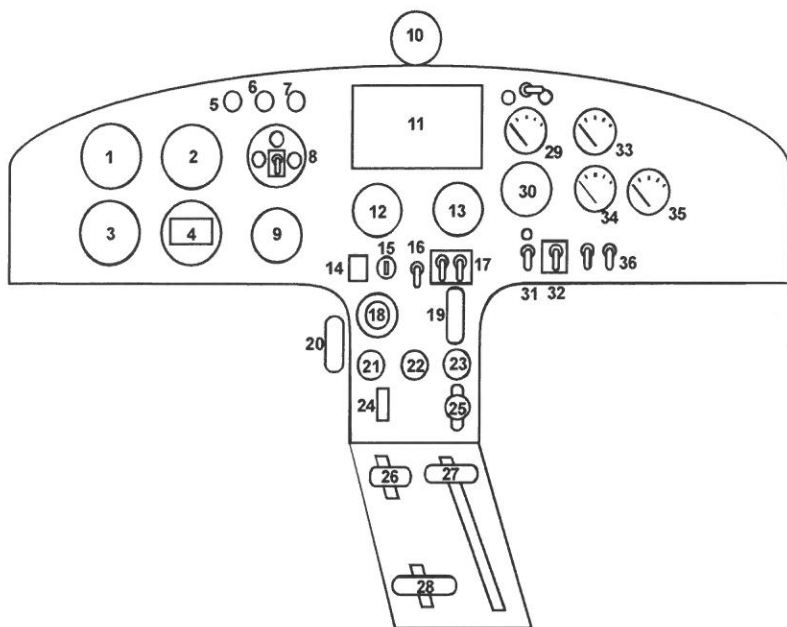
Bild 6: Bedienung und Instrumente Cockpit
