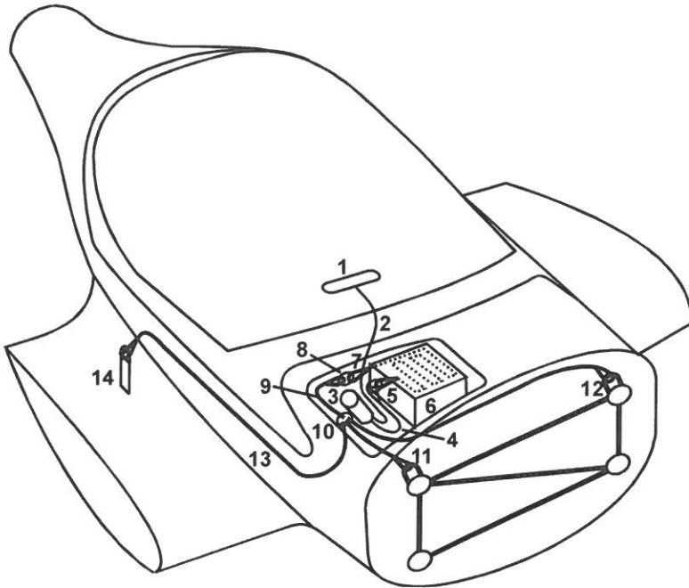
Bild 15: Einbau Rettungssystem, Rumpfansicht von links
