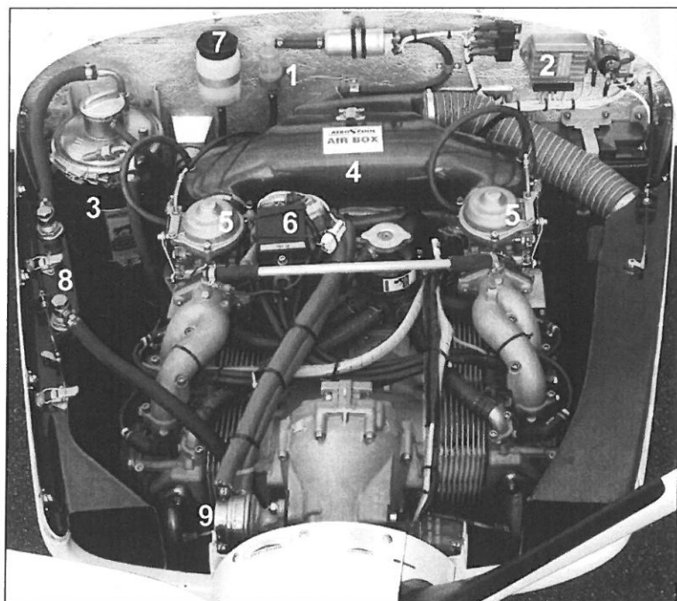
Bild 10: Triebwerk Rotax 912ULS
