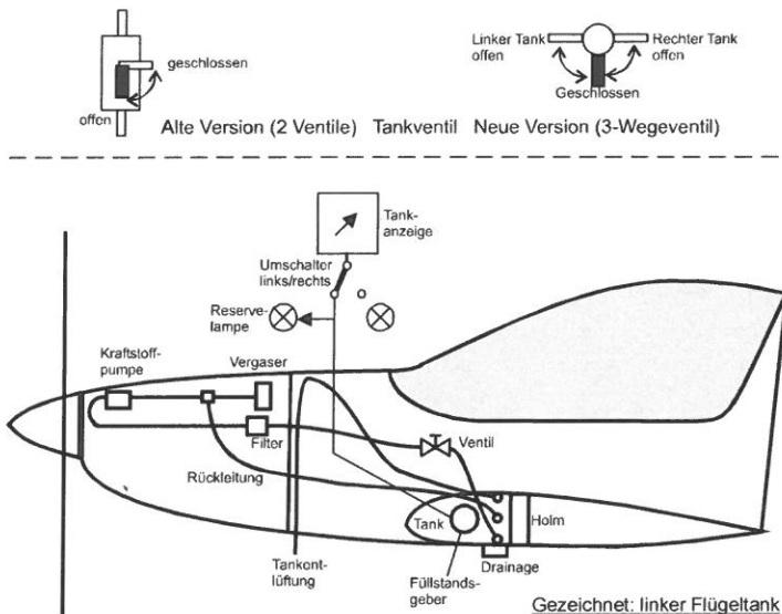
Bild 11: Prinzipskizze Kraftstoffanlage
