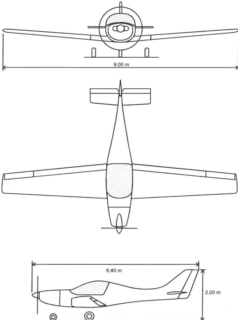
Bild 1: Dreiseitenansicht DYNAMIC mit Hauptmaßen
