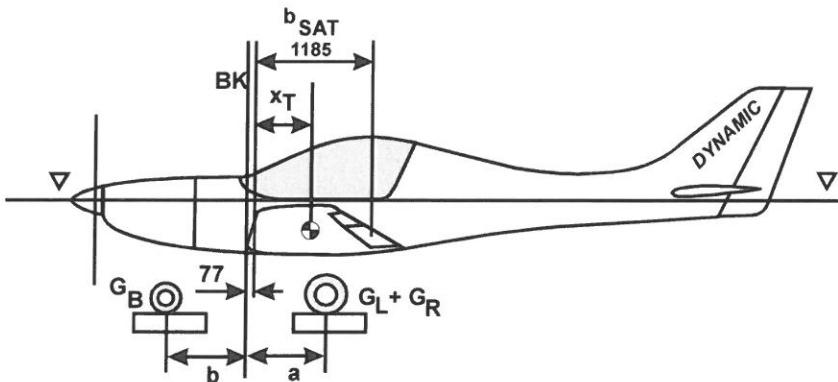
Bild 5: Schwerpunktswägung DYNAMIC
