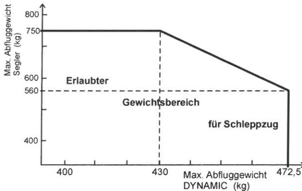
Bild 17: Zulässige Abfluggewichte Schleppzug
