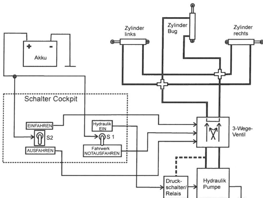
Bild 8: Funktionsprinzip Hydraulik Einziehfahrwerk
