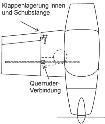
Bild 14: Lage der Verbindungen für Klappe und Querruder
