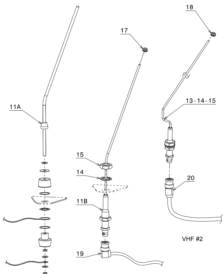
VHF
