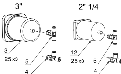
Variometer
