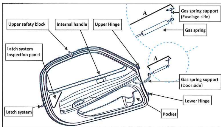
Fig. 7-6.DOOR
