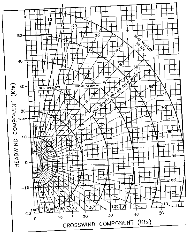
FIG. 5-2. CROSSWIND CHART
