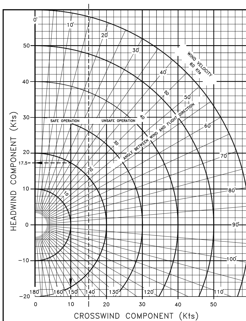
FIG. 5-2. CROSSWIND CHART
