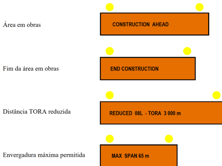
Figura E-4. Exemplos de sinalizações verticais de área fora de serviço.
