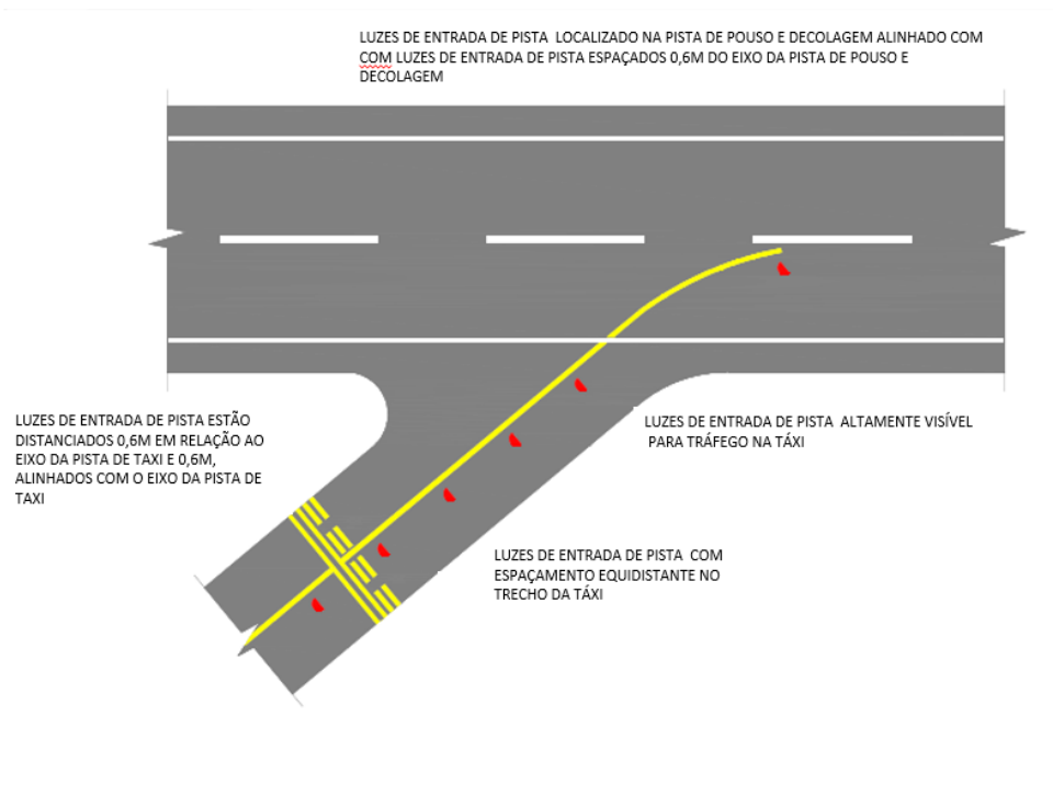
Figura D-23B. Luzes de situação de pista com táxi em ângulo
