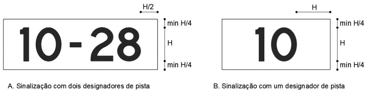
Figura AD-4. Dimensões das placas de sinalização vertical (Alterado pela Resolução nº 628, de 11.06.2021)
