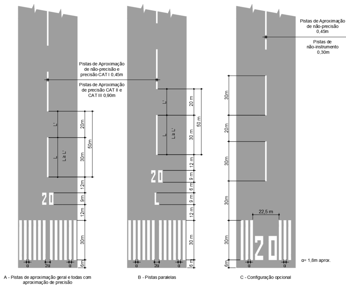
Figura D-2. Sinalização horizontal de designação de pista de pouso e decolagem, de eixo e cabeceira. (Alterada pela Resolução nº 751, de 10.07.2024)
