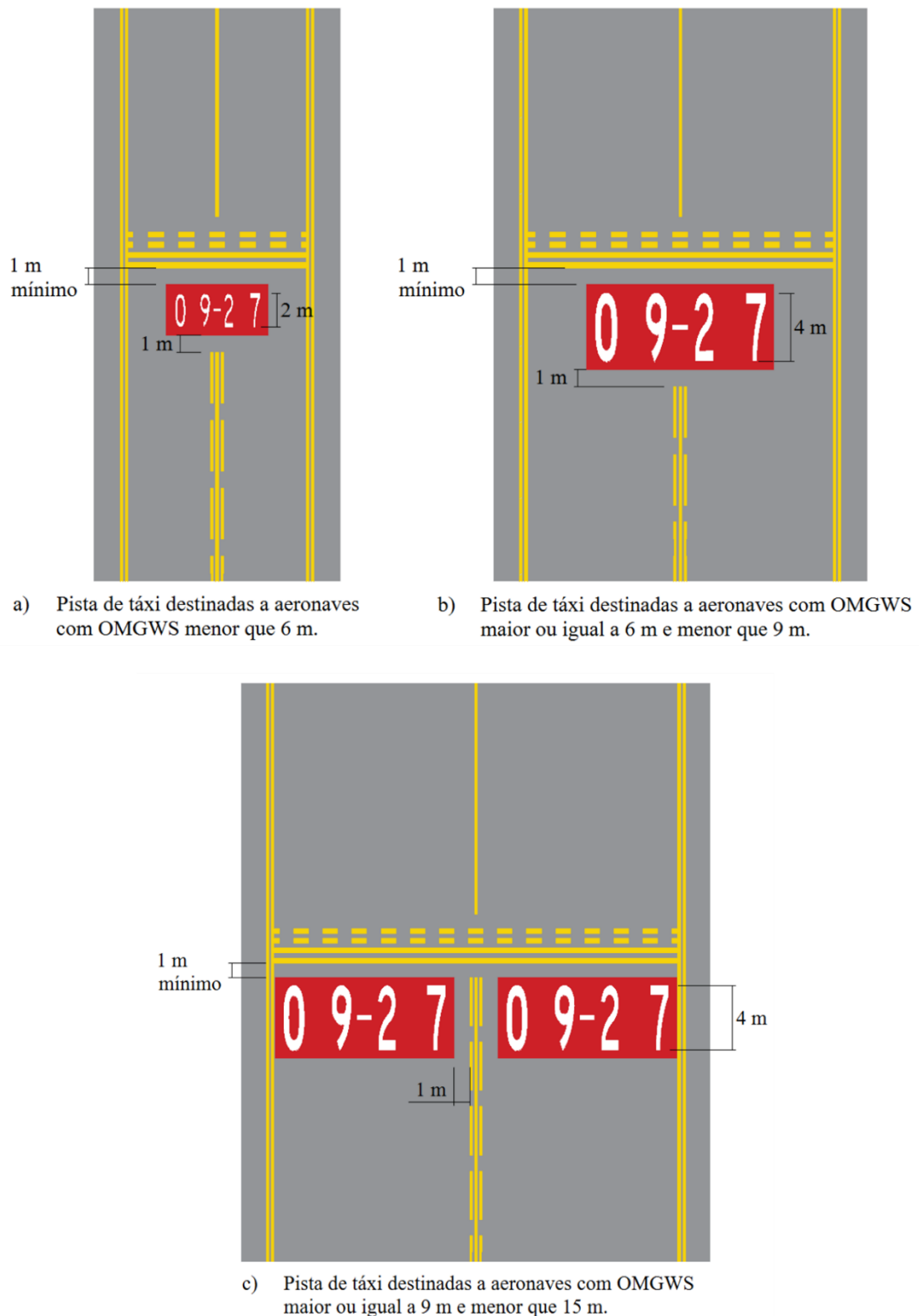
Figura D-9. Sinalização horizontal de instrução obrigatória (Alterada pela Resolução nº 802, de 18.05.2026)
