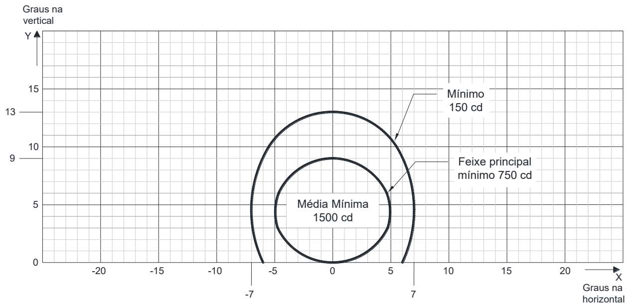
Figura AB-26. Diagrama de isocandela para luzes de espera para decolagem (THL) (luzes vermelhas)
