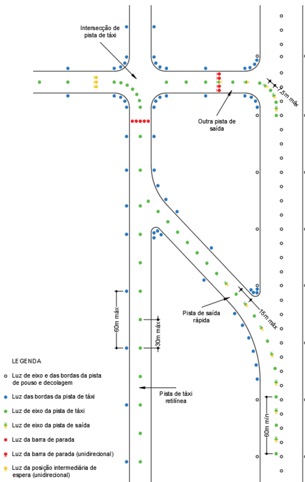
Figura D-21. Luzes de pista de taxi (Alterado pela Resolução nº 465, de 13.03.2018)
