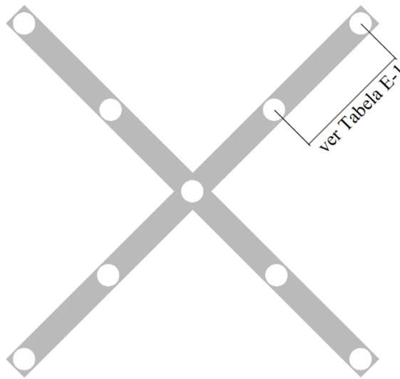
Figura E-2. Espaçamento mínimo entre eixos das luzes de pista de pouso e decolagem interditada.
