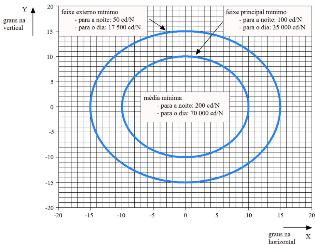
Figura AB-27. Diagrama de isocandela para luzes de pista de pouso e decolagem interditada (luz branca). (Incluída pela Resolução nº 802, de 18.05.2026)
