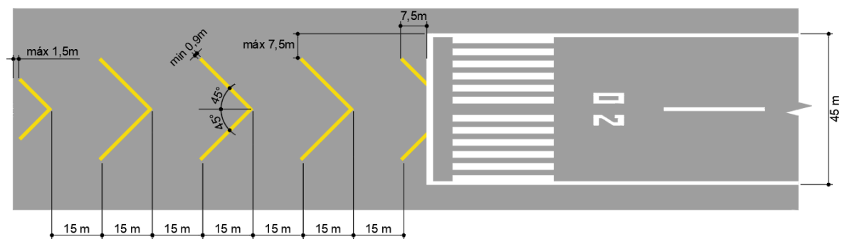
Figura E-3. Sinalização de área anterior à cabeceira. (Alterada pela Resolução nº 751, de 10.07.2024)
