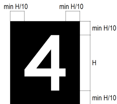
Figura AD-5. Dimensões da sinalização vertical de distância remanescente de pista (RDRS) (Incluído pela Resolução nº 802, de 18.05.2026)
