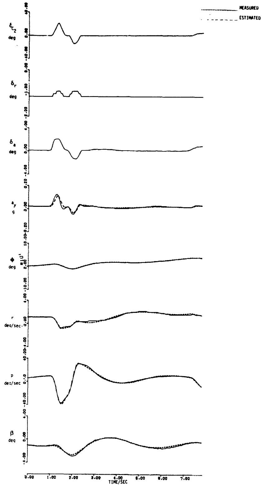
(d) Aircraft D; \delta_{z_2} pulse.
