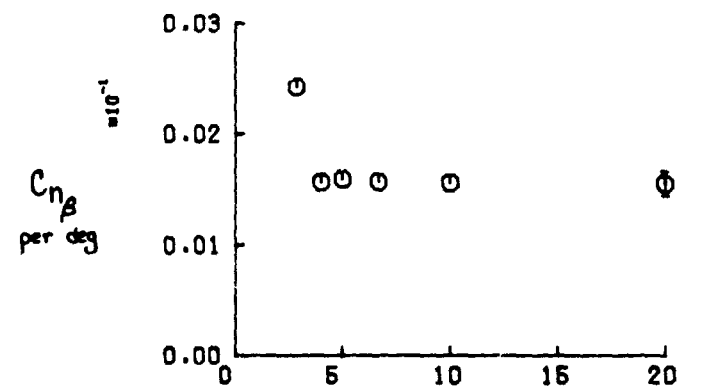
(d) C_{Y\beta} , C_{L\beta} , C_{n\beta} FOR CASE 7:17
