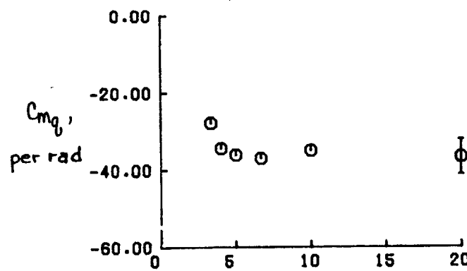
(d) C_{Z\alpha} , C_{m\alpha} , C_{mq} , FOR CASE 8.3.
